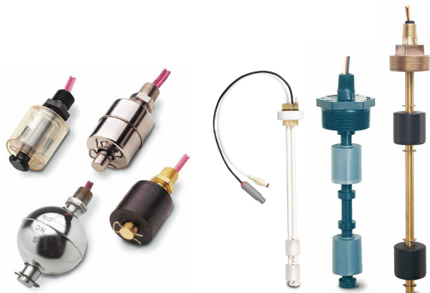
顶部或底部安装（单点式）
