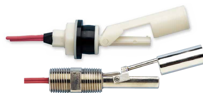
侧面安装（单点式）
